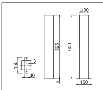
OS615 Douille à sceller
