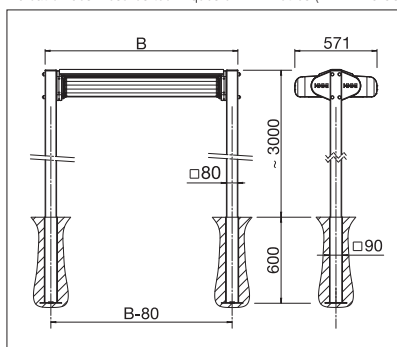
Avec douilles pour sol
