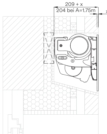
Schnitt bauseitige Blenden-Montage, Neigungswinkel 15° – 20°, hinterlüftete Fassade
