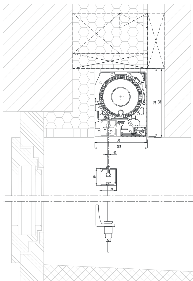
Plafondinstallatie met kabelgeleiding, doorsnede van een inbouw- en nisvariant
