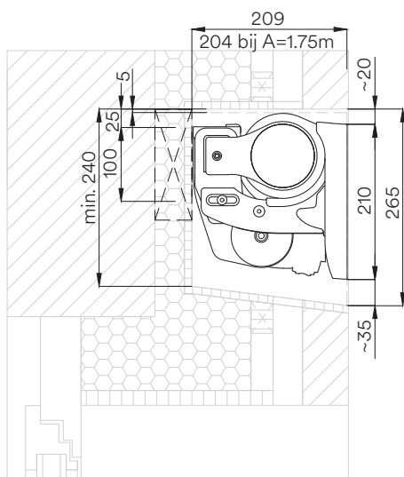
Doorsnede van een installatie- en nisvariant, hellingshoek 5° – 10°, geventileerde achtergevel
