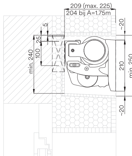
Doorsnede van een installatie- en nisvariant, hellingshoek 0° – 5°, gepleisterde gevel
