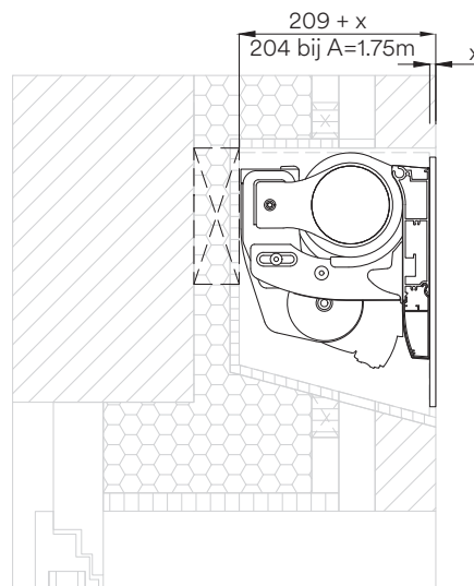
Doorsnede van paneelinstallatie op locatie, hellingshoek 15° – 20°, geventileerde achtergevel
