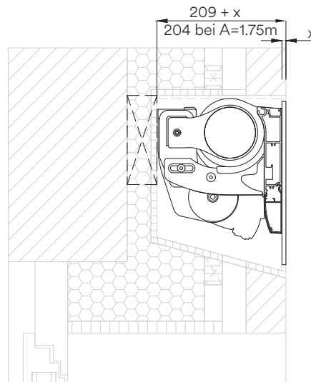
Schnitt bauseitige Blenden-Montage, Neigungswinkel 15° – 20°, hinterlüftete Fassade
