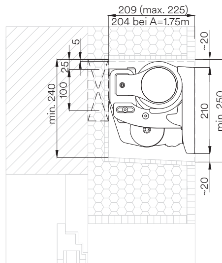
Schnitt einer Einbau- und Nischenvariante, Neigungswinkel 0° – 5°, verputzte Fassade
