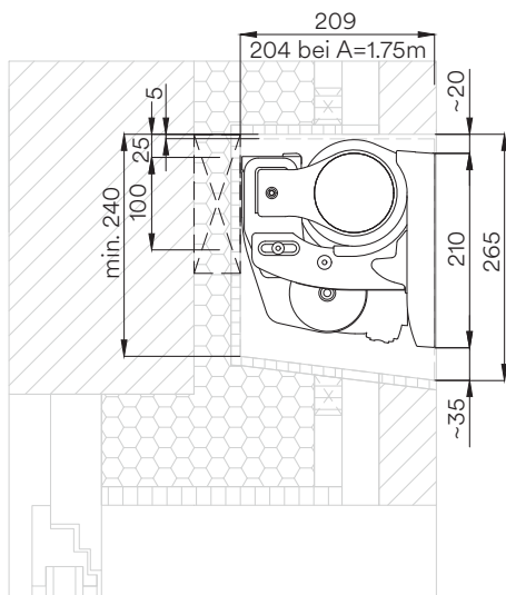
Schnitt einer Einbau- und Nischen-Variante, Neigungswinkel 5° – 10°, hinterlüftete Fassade
