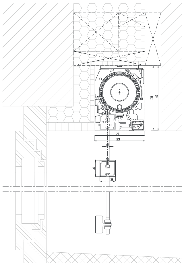
Deckenmontage mit Stangenführung, Schnitt einer Einbau- und Nischen-Variante
