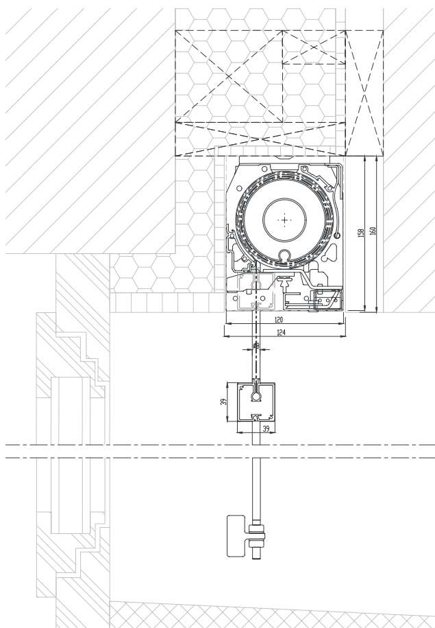
Installazione a soffitto con guida tondino, Sezione di una variante d'installazione e di nicchia
