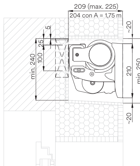
Sezione di una variante d'installazione e di nicchia, angolo di inclinazione 0° – 5°, facciata intonacata
