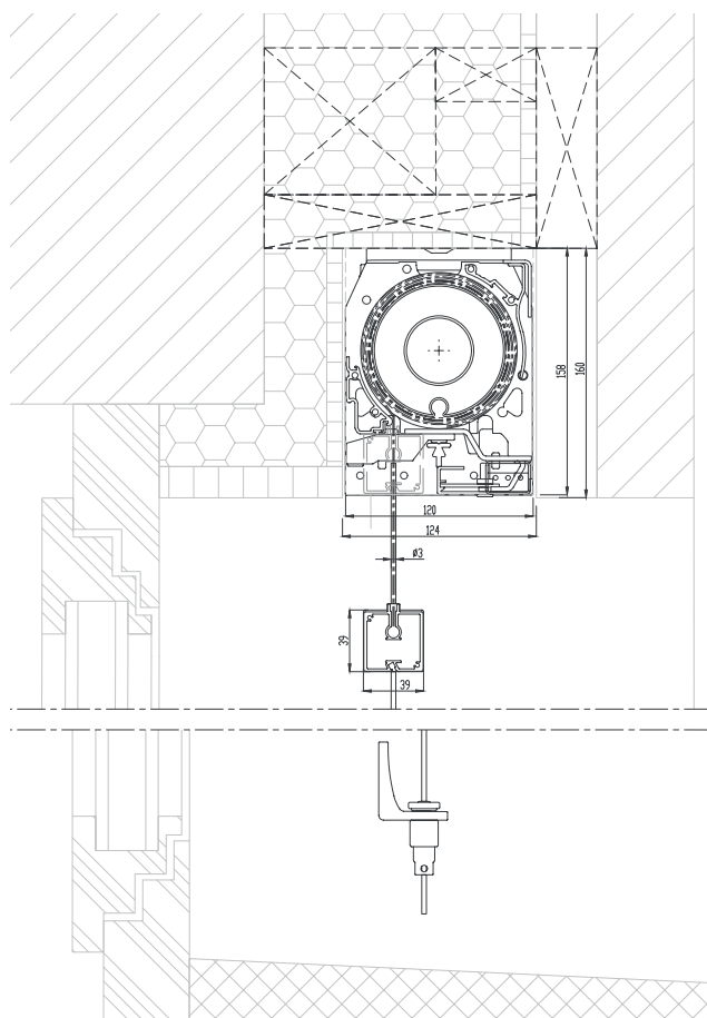
Installazione a soffitto con guida a cavetto, Sezione di una variante d'installazione e di nicchia
