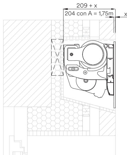
Vista in sezione dell'installazione dei pannelli in loco, angolo di inclinazione 15° – 20°, facciata retroventilata
