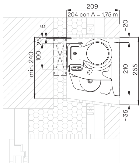
Sezione di una variante d'installazione e di nicchia, angolo di inclinazione 5° – 10°, facciata retroventilata
