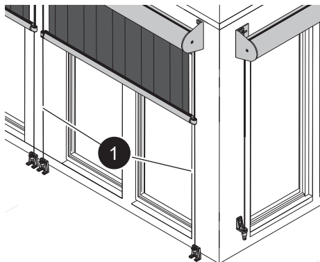
Fig. 10: Cable guide
